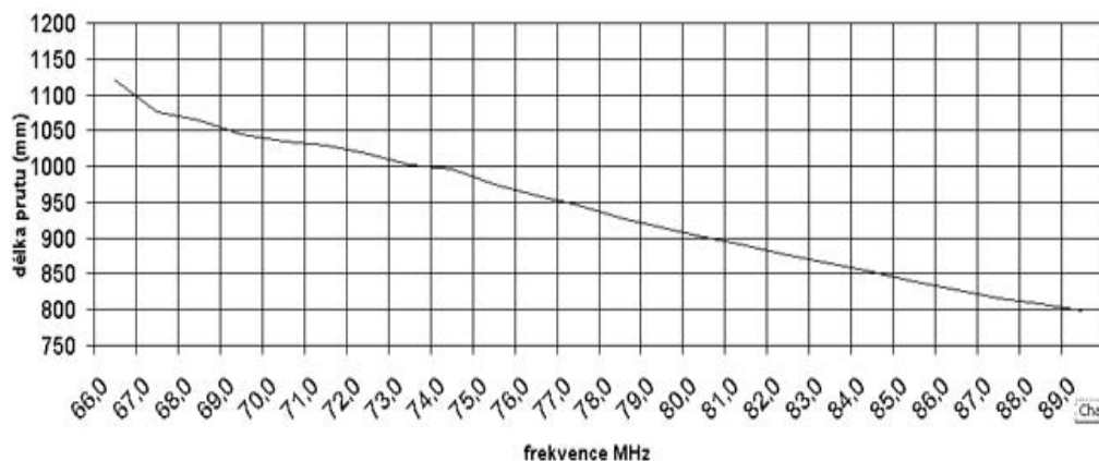
Diagram zkrácení PVA 001
