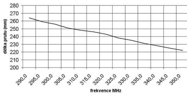
Diagram zkrácení PVA 001 - 330MHz
