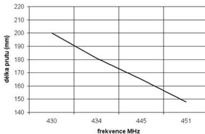
Diagram zkrácení PVA 001 - 440MHz
