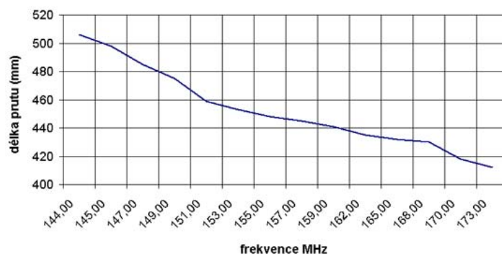
Diagram zkrácení PVA 001 - 160MHz
